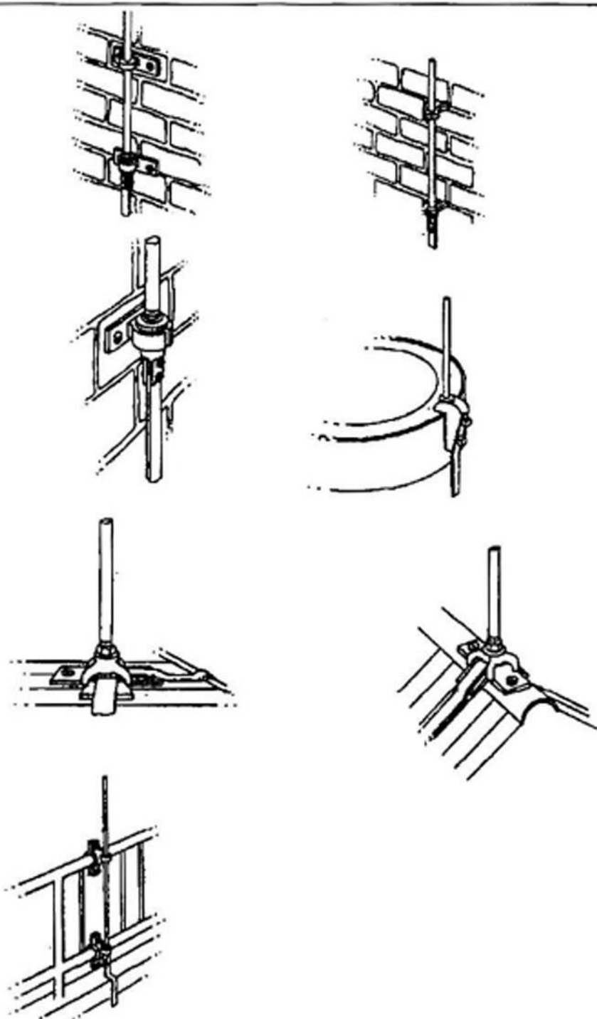
Hình 8 - Các kiểu kìm thu sét điện hình
