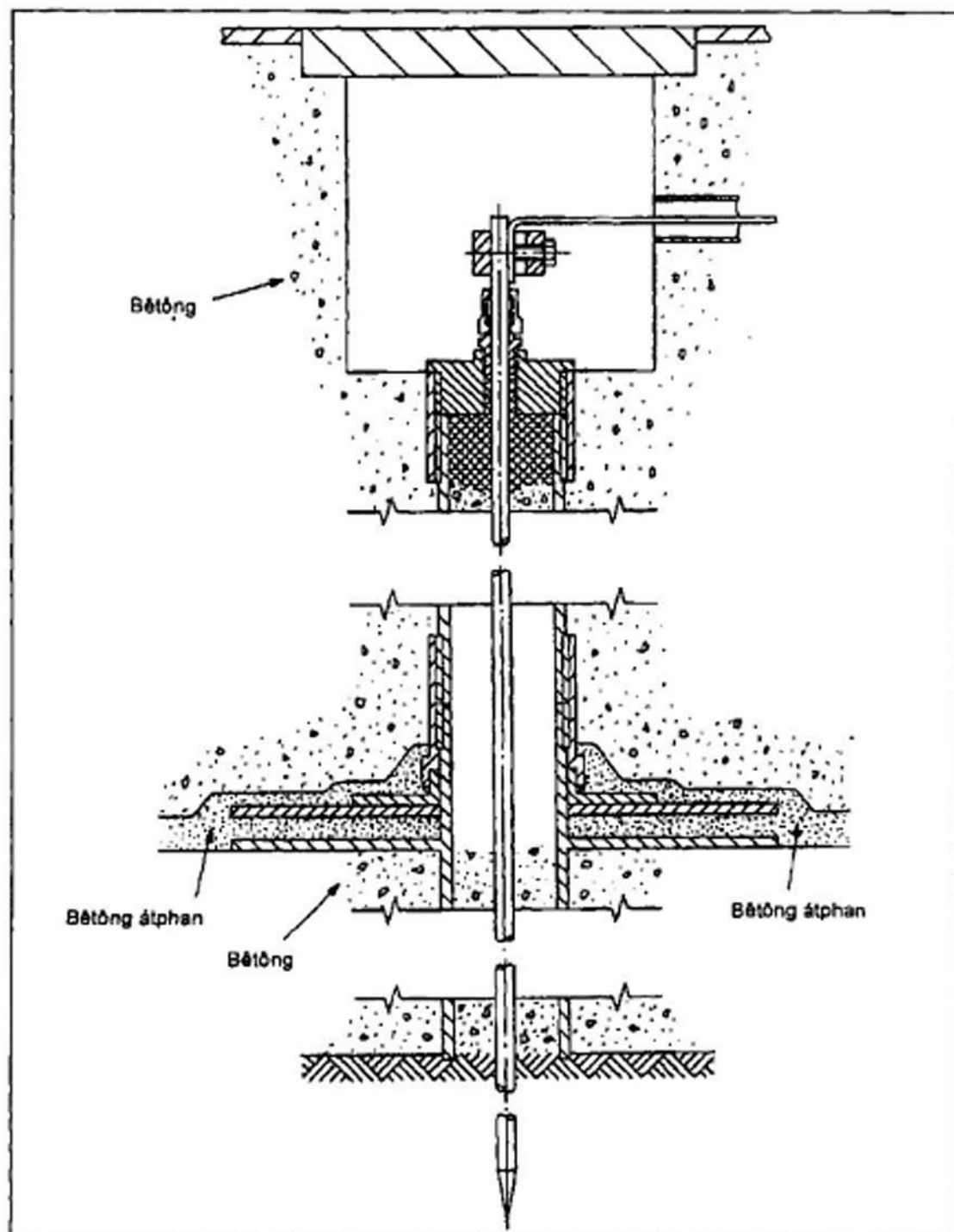
Hình 23 - Ví dụ về cọc nổi đất có lớp bọc được sử dụng trong kết cấu bê chứa
